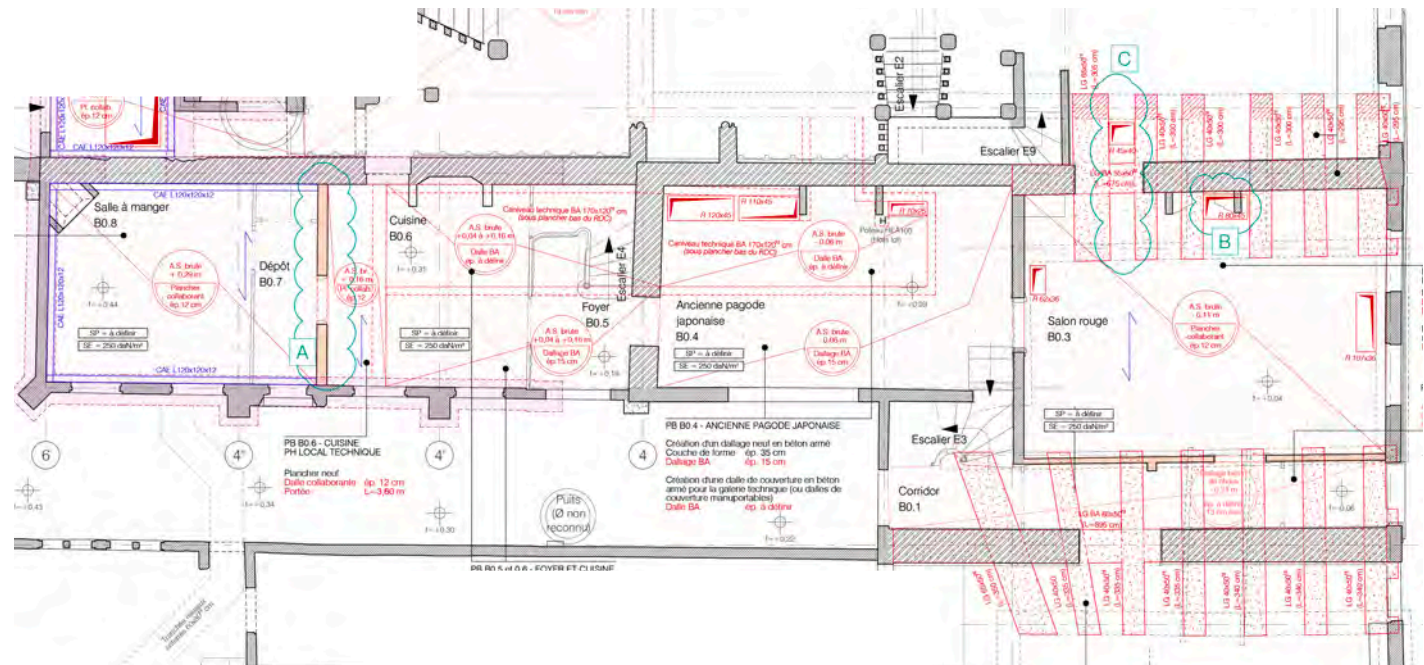
Plan des reprises de fondations.
